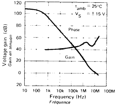
OPEN LOOP FREQUENCY RESPONSE REPONSE EN FREQUENCE EN BOUCLE OUVERTE
