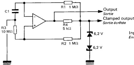
LF SQUARE WAVE GENERATOR GENERA TEUR DE SIGNAUX CARRES BF
